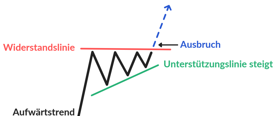
Steigendes Dreieck-Muster
