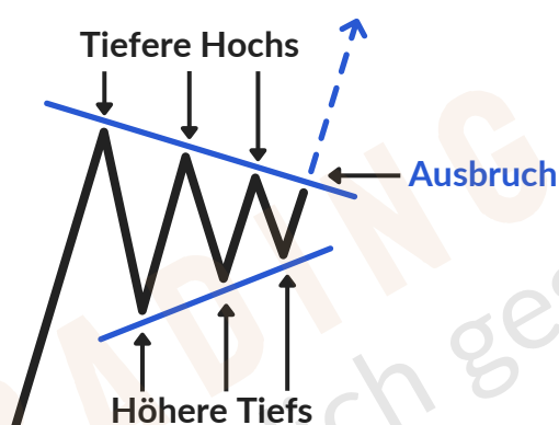
Symmetrisches Dreieck-Muster
